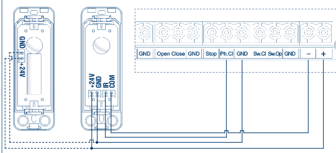
Рис./Fig. 18. SHAFT-60/120/150/200/500/1000
