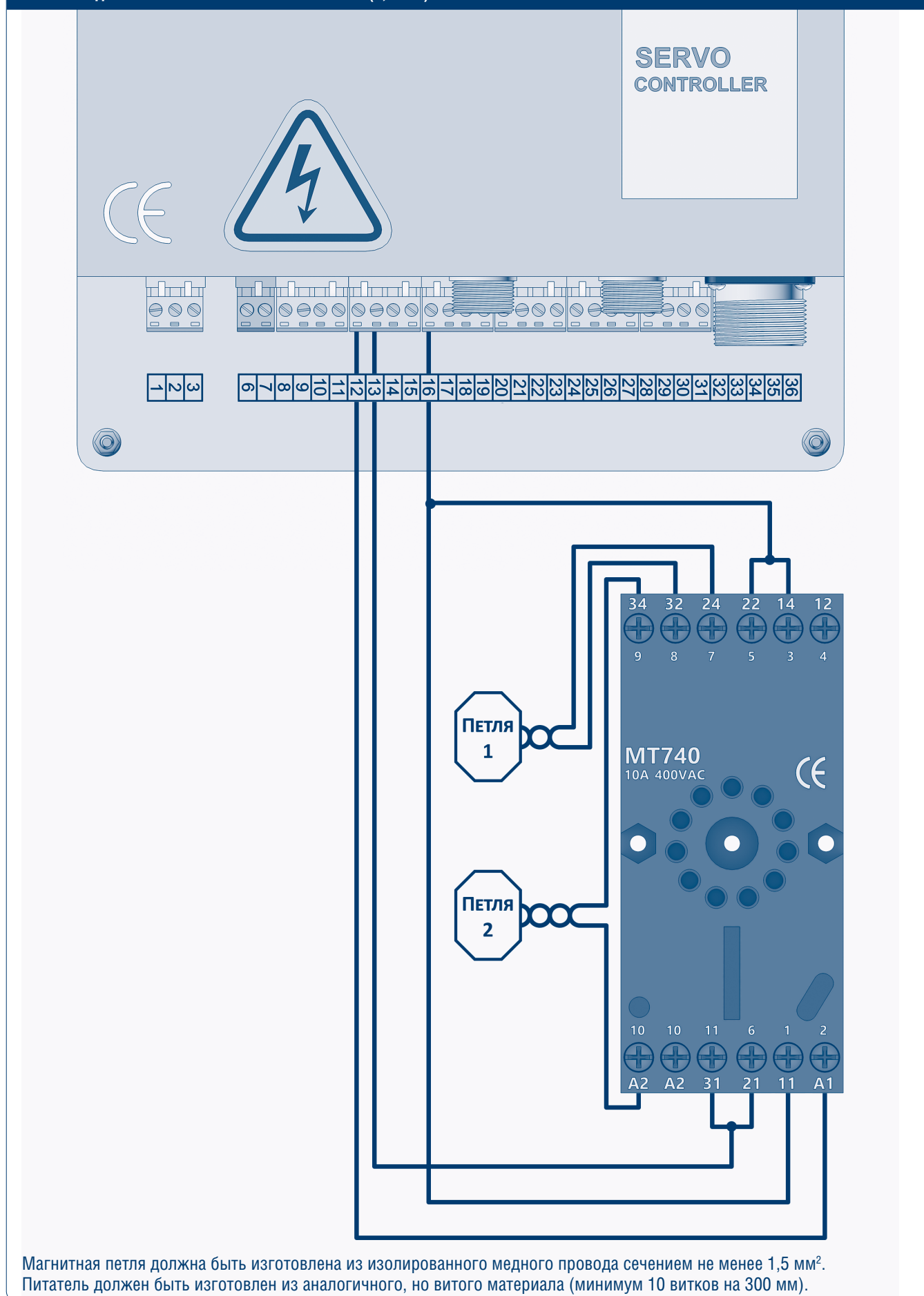
Рис. 11. Подключение магнитной петли LOOP-2 (1,5 кВт)
