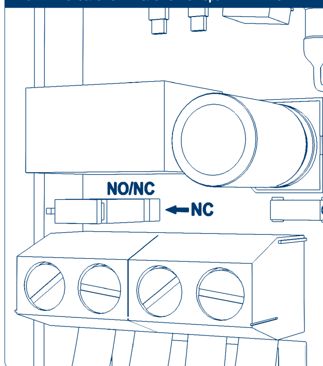
Рис. 21. Фотозлемент. Положение переключки — NC
