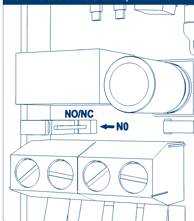
Рис. 22. Фотозлемент. Положение переключки — NO
