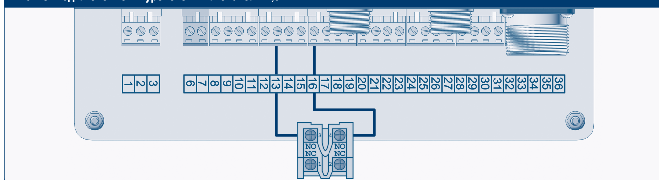
Рис. 18. Подключение шнуrowого выключателя 1,5 кВт
