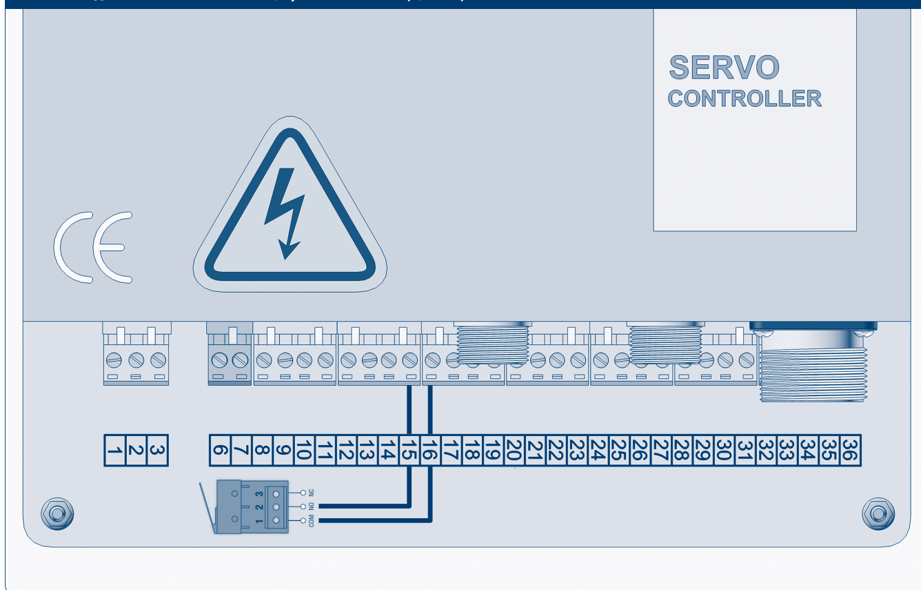
Рис. 13. Подключение ключ-кнопки, арт. KEYSWITCH (1,5 кВт)
