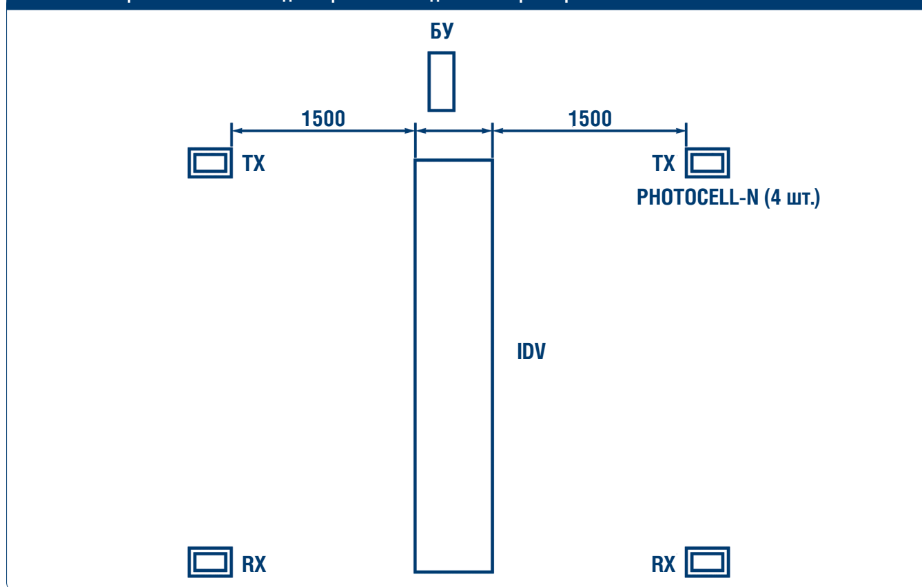
Рис. 20. Схема расположения стоек для вертикально-подъемных ворот серии IDV
