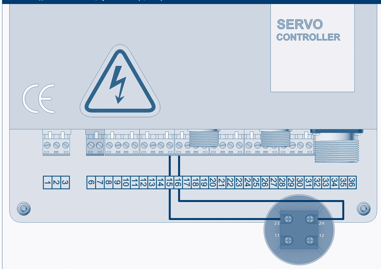
Рис. 12. Подключение кнопки, арт. DKN009 (1,5 кВт)
