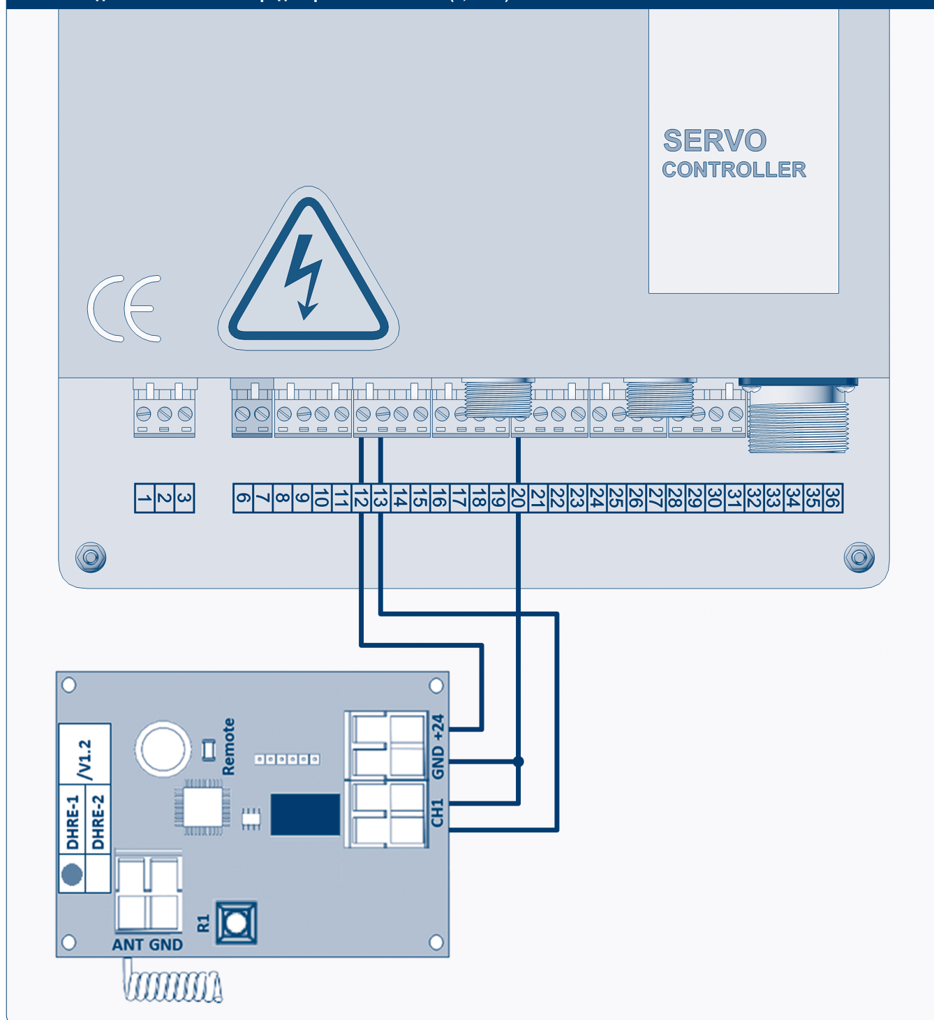
Рис. 17. Подключение внешнего радиоприемника DHRE-1 (1,5 кВт)
